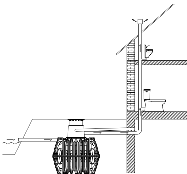
Desaireación con salida libre
