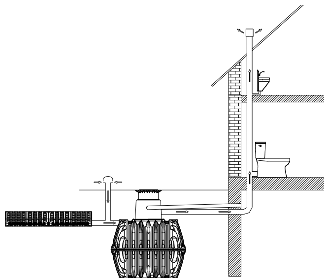
Entlüftung bei Versickerung oder nicht freiem Ablauf
