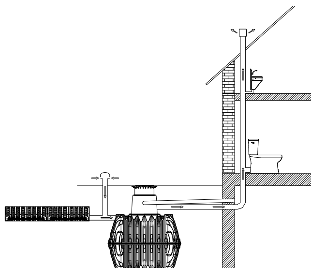
Desaireación en caso de filtración de agua de lluvia o salida restringida
